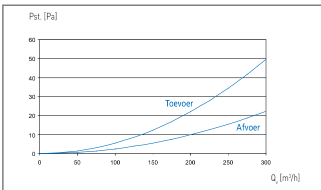
Weerstand ventilatiedakdoorvoer, D160 geïsoleerd (toevoer en afvoer)
