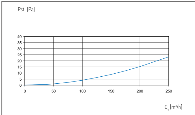
Weerstand ventilatietoever (onder pannen), D160 geïsoleerd
