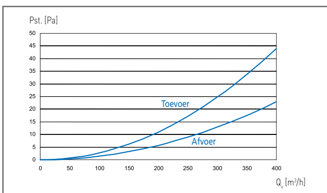
Weerstand ventilatiedakdoorvoer, D180 geïsoleerd (toevoer en afvoer)
