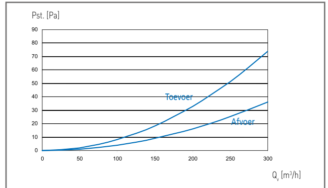
Weerstand ventilatietoever (onder pannen), D125 geïsoleerd
