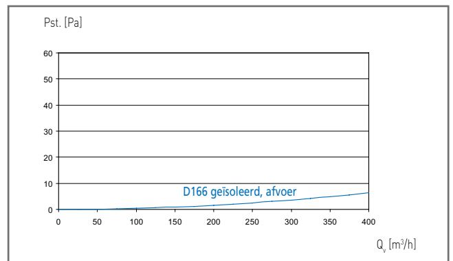
Weerstand ventilatiedakdoorvoer, D166 geïsoleerd (afvoer)
